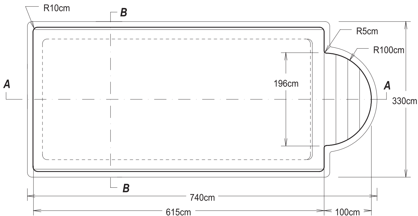
Grundplan
