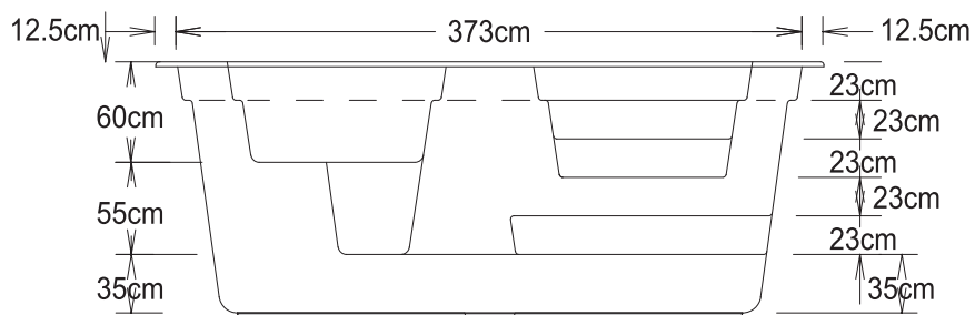
Sektion B - B
